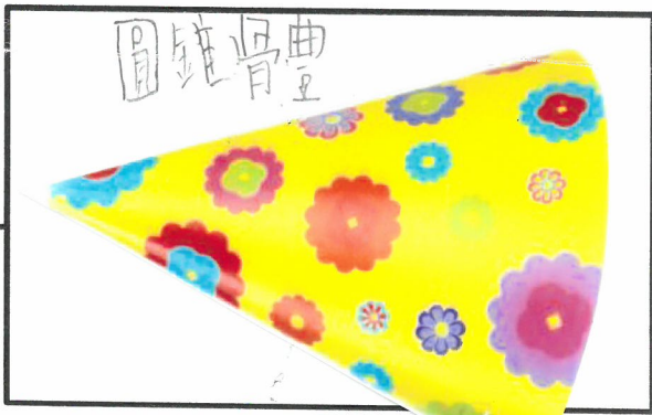
圓錐體
